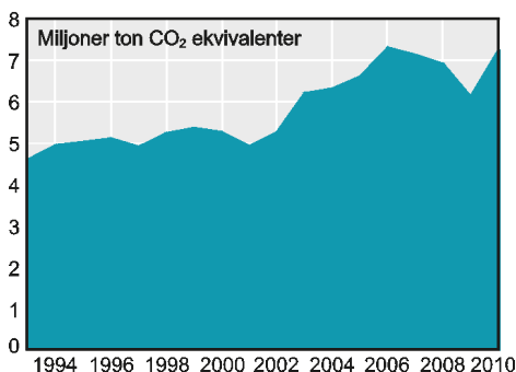
Utsläpp av växthusgaser till följd av svensk konsumtion, 1993–2010, miljoner ton CO 2 -ekvivalenter
